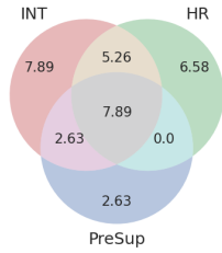
(d) EMH
