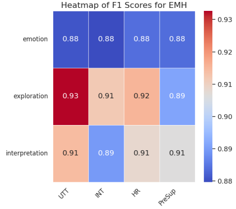
(d) EMH
