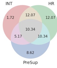
(b) P4G
