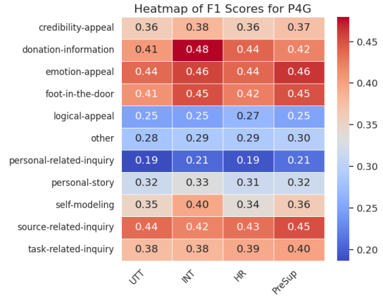
(b) P4G
